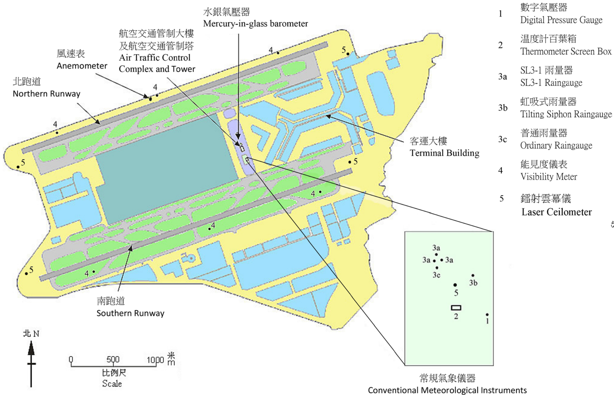
圖 4 香港國際機場航空氣象儀器分布圖 (二零一七年十二月三十一日)
