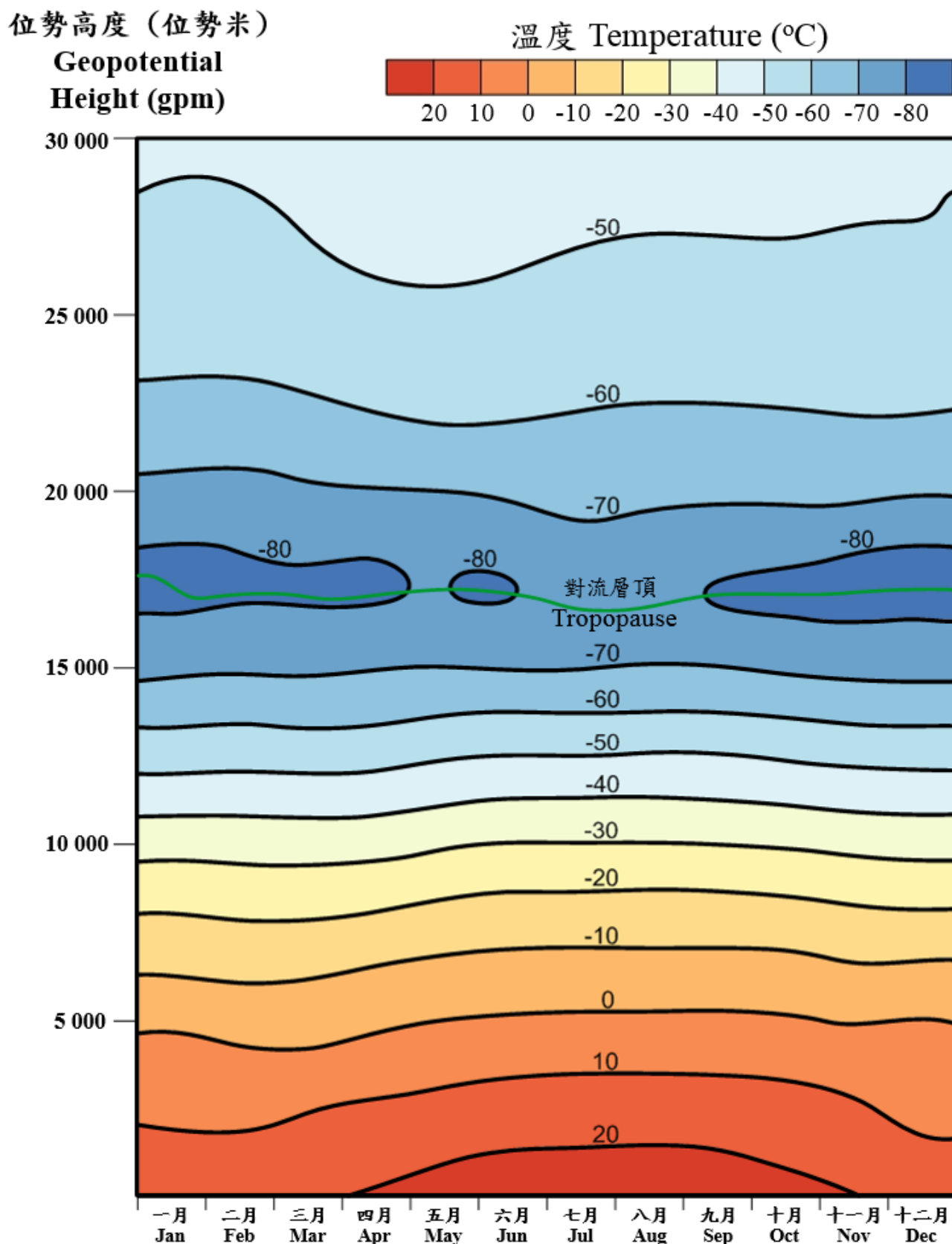
圖 14 各位勢高度於二零一七年協調世界時零時的月平均溫度
