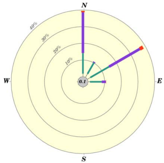
圖 7 (續) 橫瀾島於二零一七年每月的風玫瑰圖(七月至十二月)
