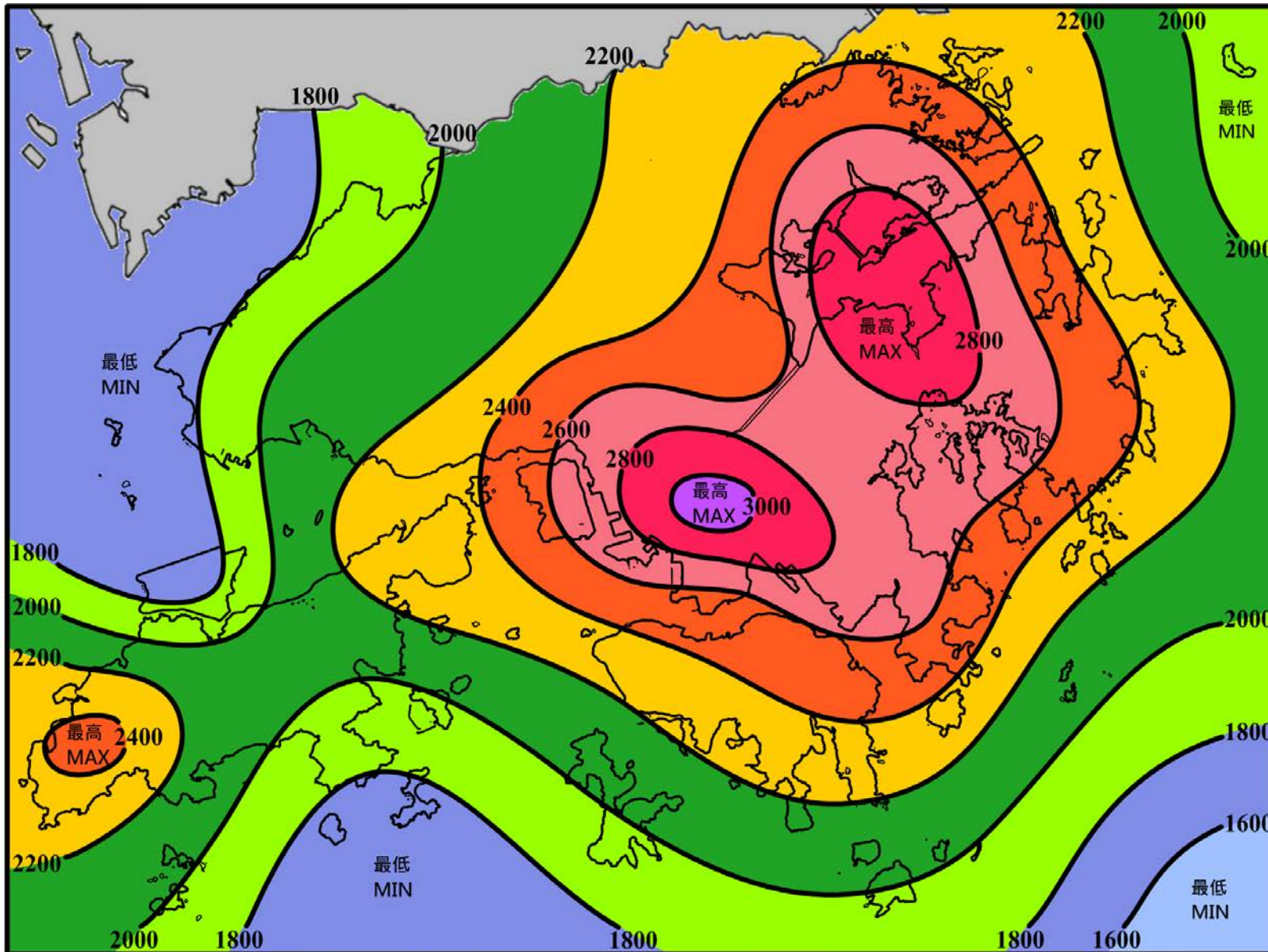
圖 12 二零一七年全年雨量分布圖 (等雨量線單位為毫米)
