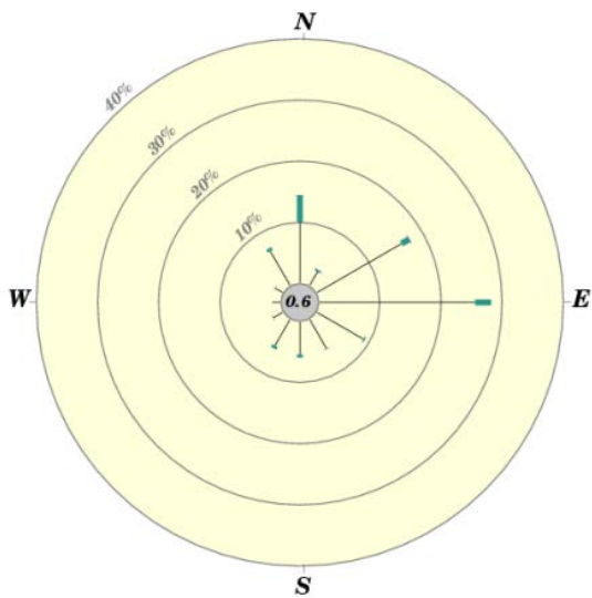
圖 8 自動氣象站於二零一七年的年風玫瑰圖
