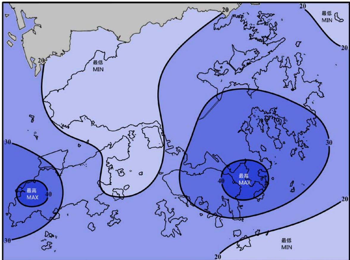
圖 11 (續) 二零一七年十一月的雨量圖 (等雨量線單位為毫米)
