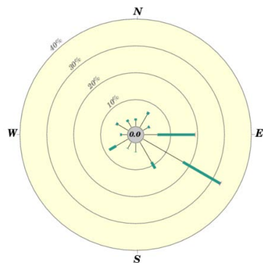
圖 8 (續) 自動氣象站於二零一七年的年風玫瑰圖
