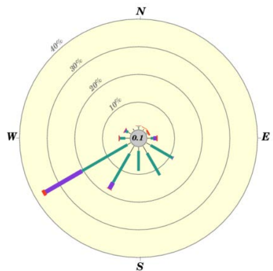
圖 7 橫瀾島於二零一七年每月的風玫瑰圖(一月至六月)
