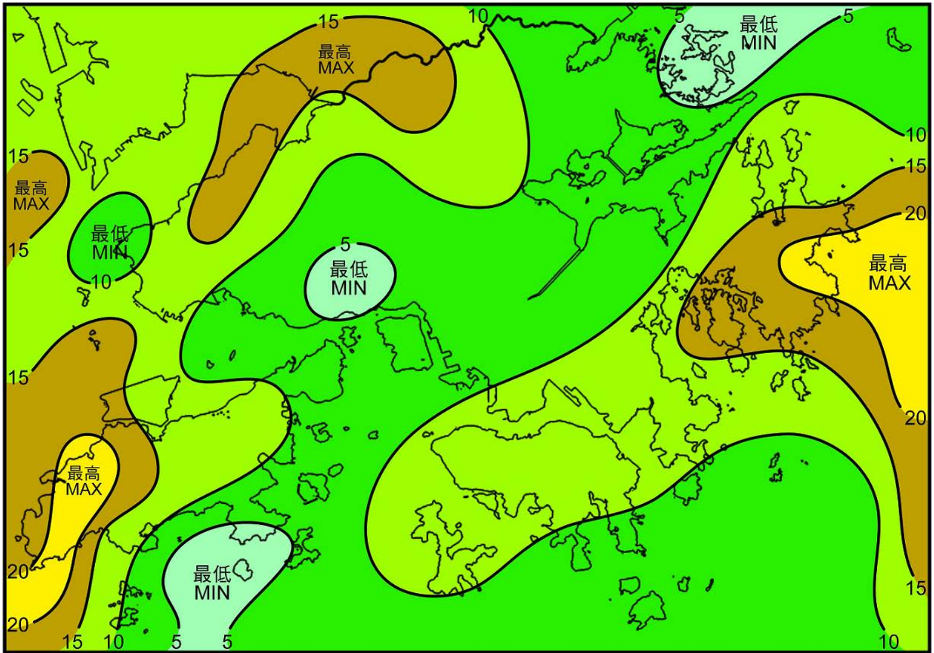
圖 16 二零一七年全年雲對地閃電密度圖 (等值線單位為每年每平方公里閃電次數)
