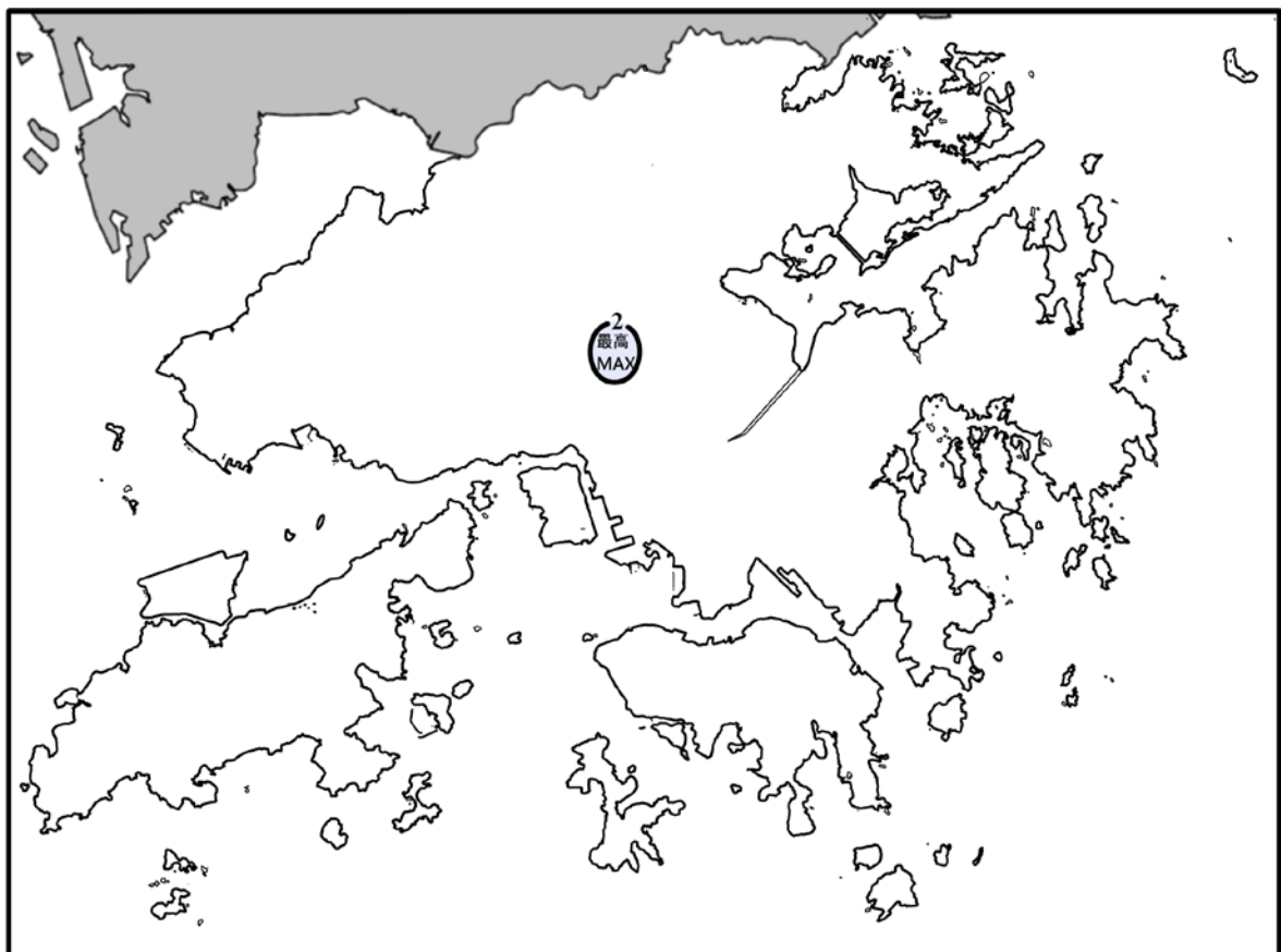
圖 11 (續) 二零一七年十二月的雨量圖 (等雨量線單位為毫米)
