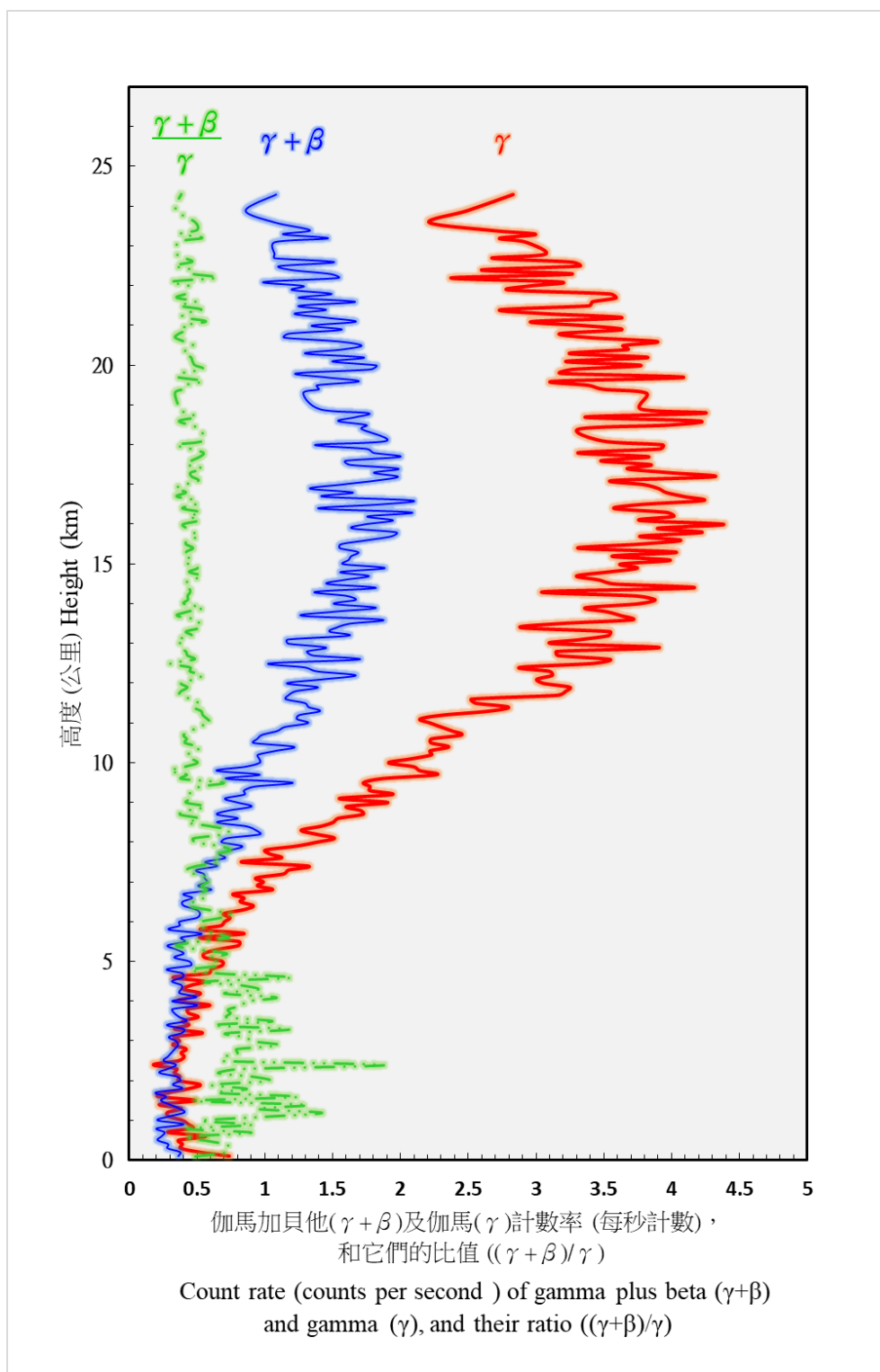
圖 7. 二零二五年內在京士柏進行的高空輻射探測之平均大氣放射性垂直廓線 (探測日期為：十月二十七日、十一月十四日及十二月二十四日)。
