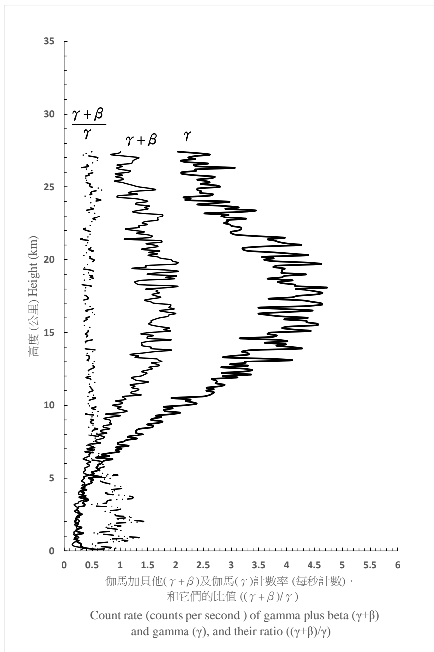
圖 7. 二零一八年內在京士柏進行的高空輻射探測之平均大氣放射性垂直廓線 (探測日期為：二月二十六日、三月二十九日、六月二十一日、十月八日、十一月八日)。
