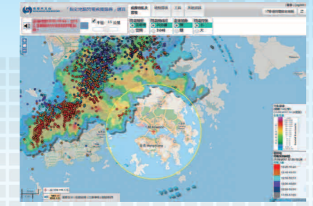
實時閃電位置分佈及戒備範圍 (圖圈)
