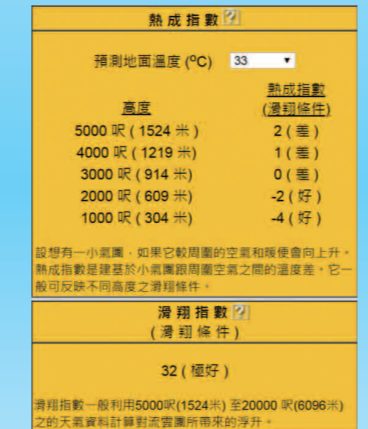
在不同高度的熱成指數和滑翔指數預測
