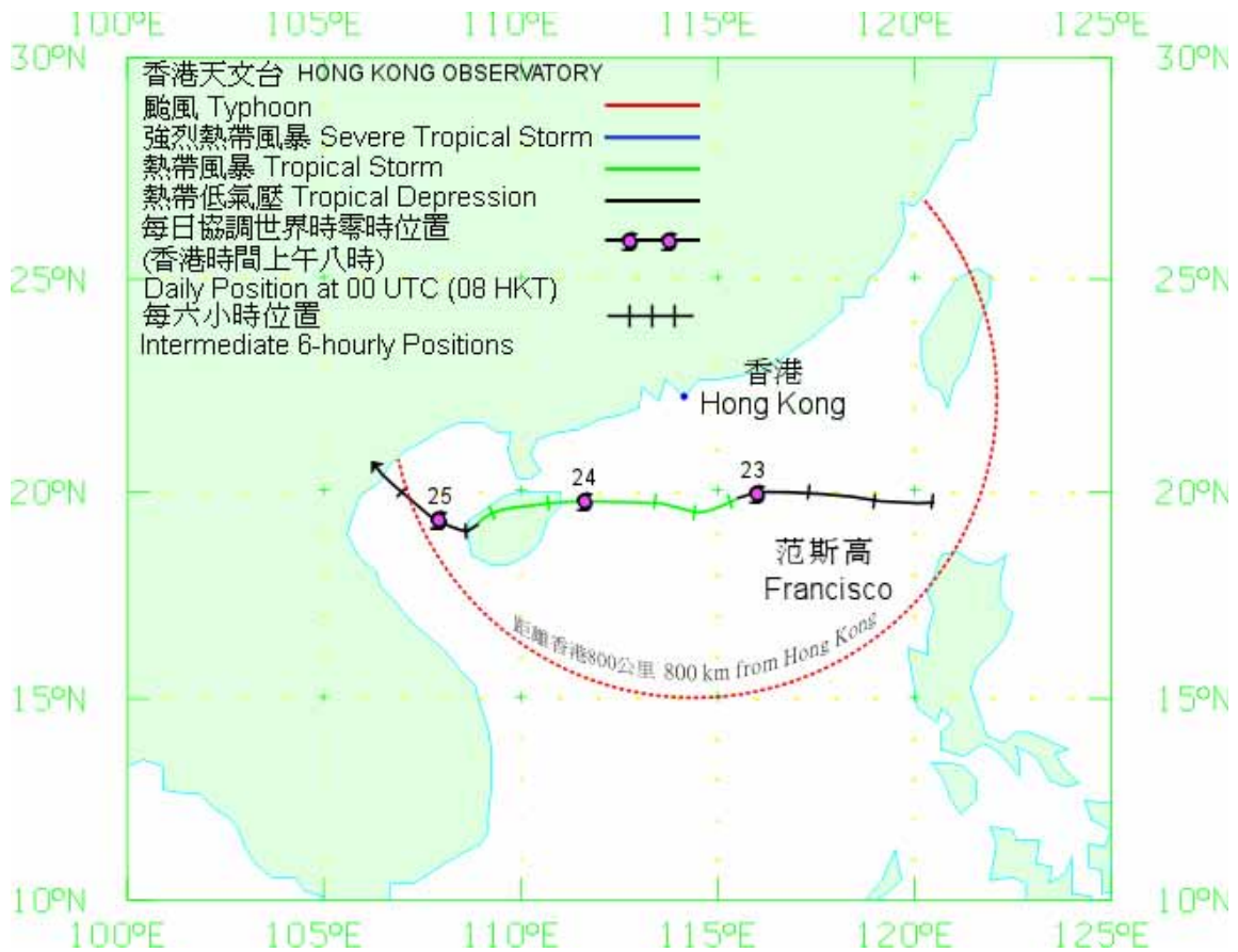
圖 3.2.1 范斯高 (0713) 在二零零七年九月二十二日至二十六日的路徑圖。 Figure 3.2.1 Track of Francisco (0713) on 22 – 26 September 2007.
