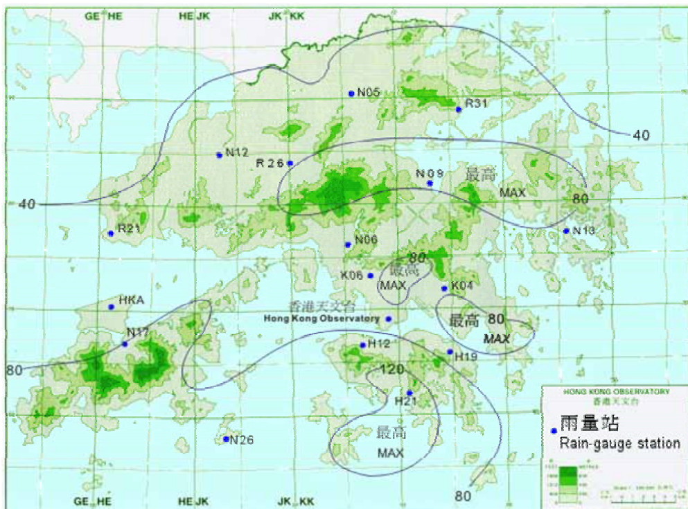
圖 3.2.2 二零零七年九月二十三日至二十四日的雨量分佈(等雨量線單位為毫米)。 Figure 3.2.2 Rainfall distribution on 23 – 24 September 2007 (isohyets are in millimetres).
