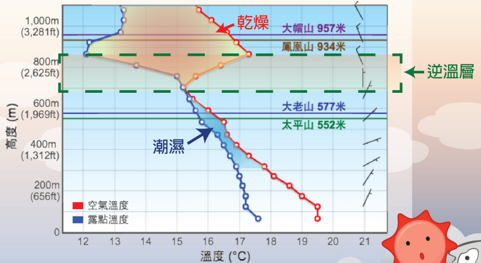
空氣溫度、露點溫度、風速及風向的垂直高度 (0 - 1,000米) 變化
