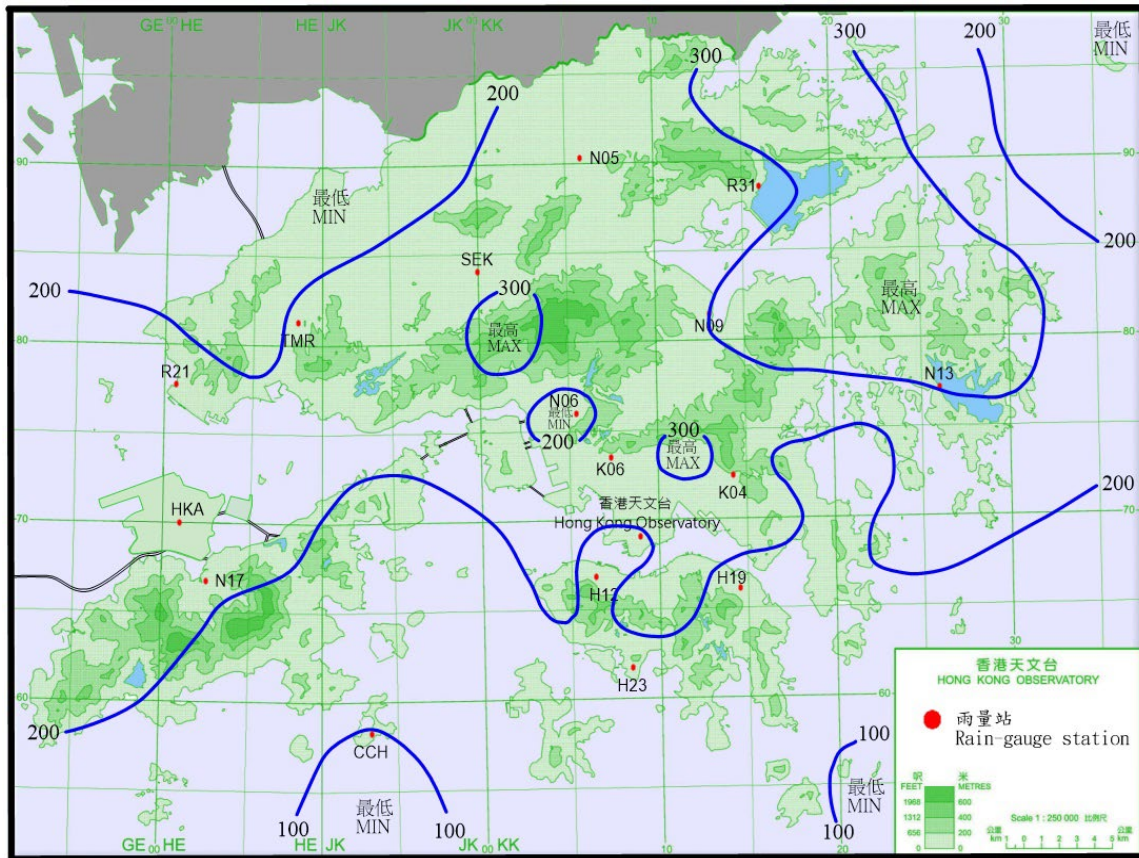
圖 3.11.3 二零二五年九月二十二日至二十五日的雨量分佈(等雨量線單位為毫米)。 Figure 3.11.3 Rainfall distribution on 22 – 25 September 2025 (isohyets are in millimetres).
