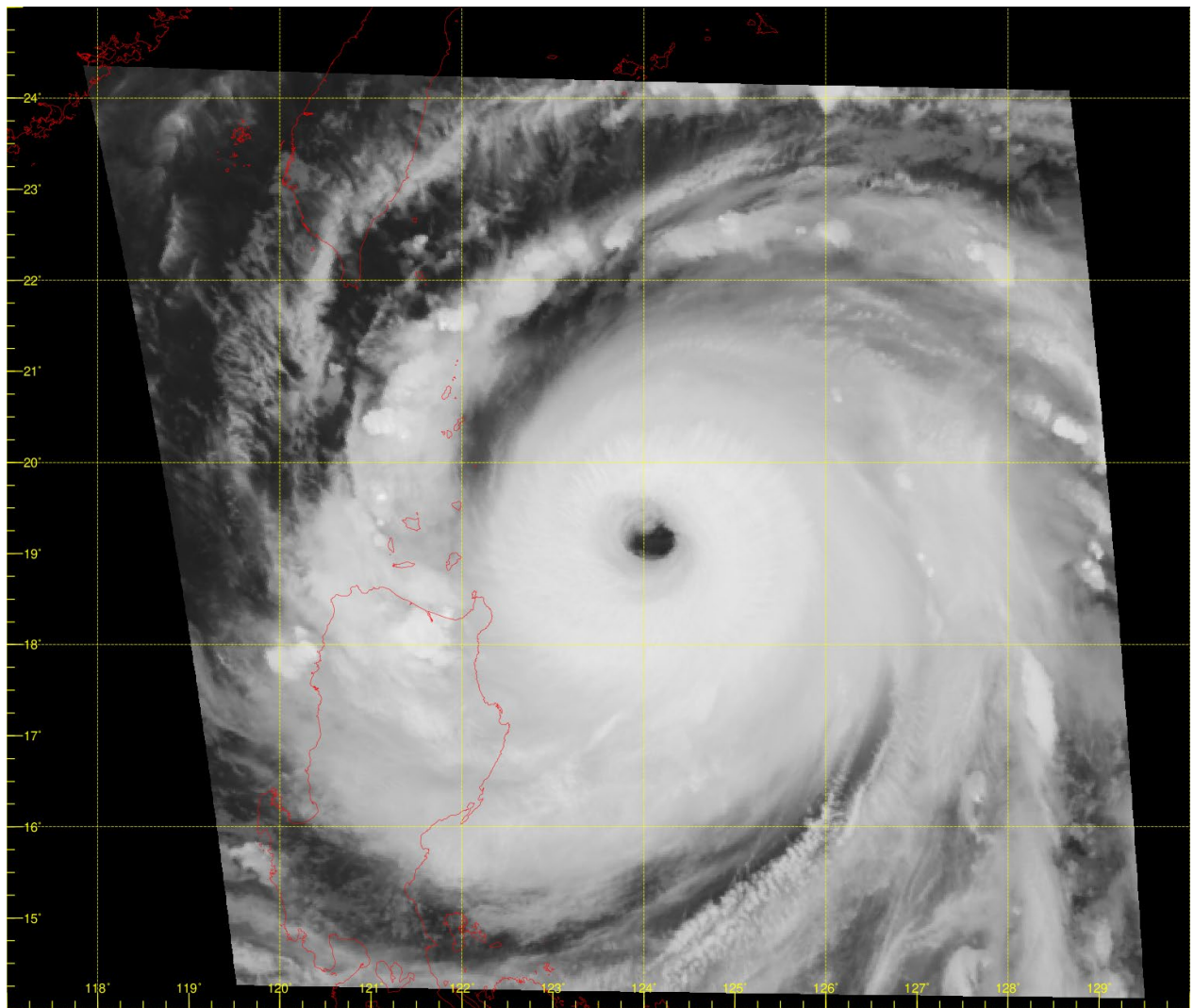
圖 2.3 二零二五年九月二十二日上午2時左右超強颱風樺加沙(2518)的紅外線衛星圖片，當時樺加沙達到其最高強度，中心附近最高持續風速估計為每小時230公里，而最低海平面氣壓為905百帕斯卡。
