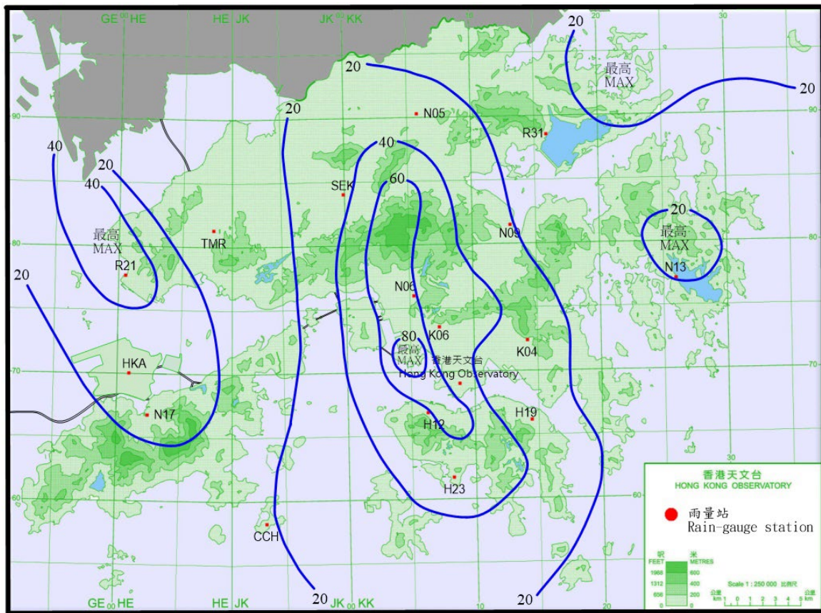
圖 3.2.2 二零二五年六月二十五日至二十六日的雨量分佈(等雨量線單位為毫米)。 Figure 3.2.2 Rainfall distribution on 25 – 26 June 2025 (isohyets are in millimetres).
