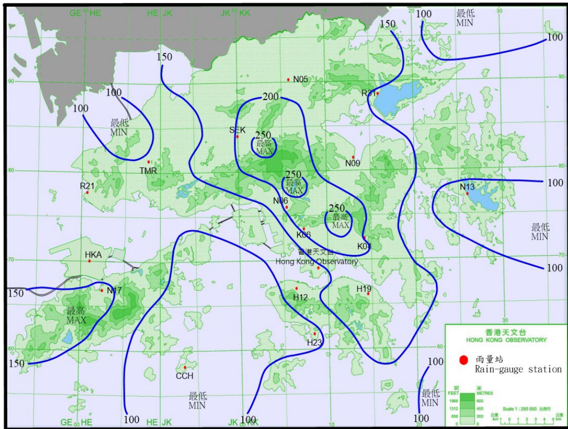
圖 3.4.3 二零二五年七月十九日至二十一日之雨量分佈(等雨量線單位為毫米)。 Figure 3.4.3 Rainfall distribution on 19 – 21 July 2025 (isohyets are in millimetres).
