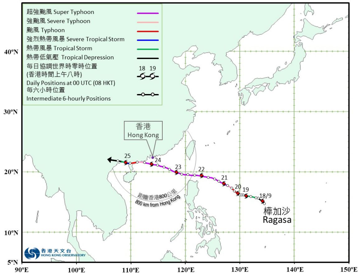
圖 3.11.1a 二零二五年九月十八日至二十五日樺加沙(2518)的路徑圖。
