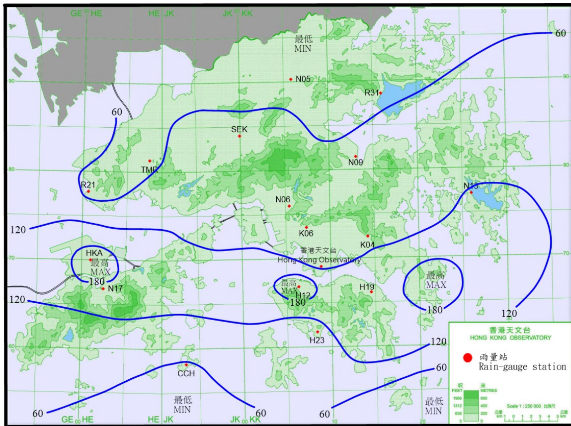
圖 3.10.2 二零二五年九月十七日至二十日的雨量分佈(等雨量線單位為毫米)。 Figure 3.10.2 Rainfall distribution on 17 – 20 September 2025 (isohyets are in millimetres).
