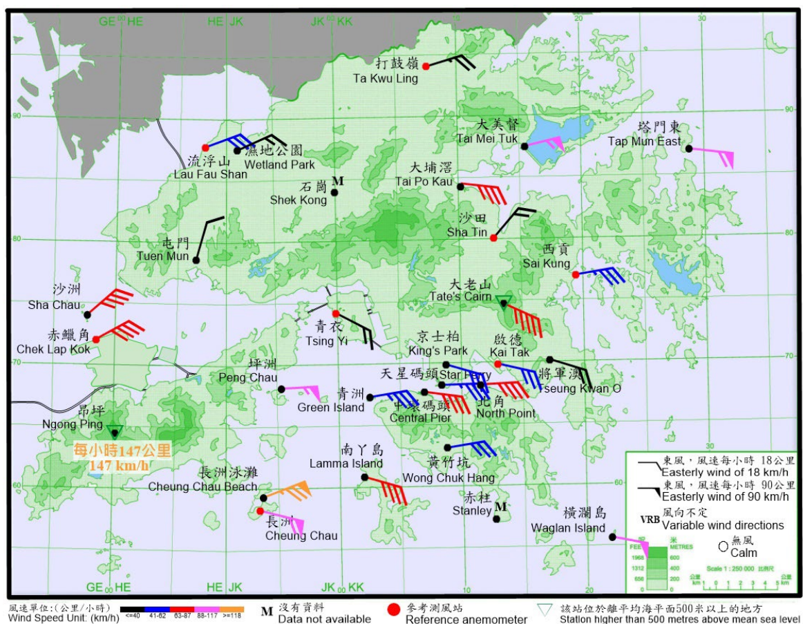
圖 3.4.6b 二零二五年七月二十日上午11時35分香港各站錄得的十分鐘平均風向和風速。當時本港普遍吹偏東風，長洲泳灘及昂坪的風力達到颶風程度。
