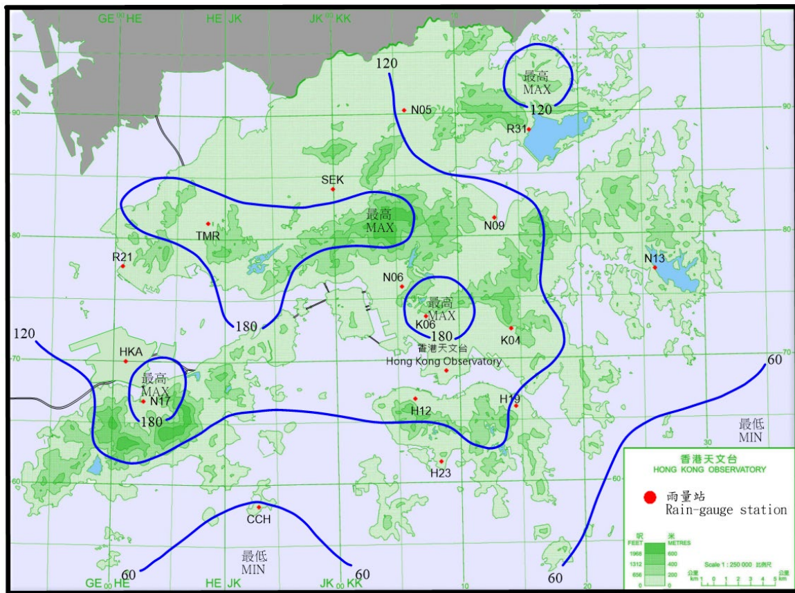
圖 3.9.2 二零二五年九月五日至九日的雨量分佈(等雨量線單位為毫米)。 Figure 3.9.2 Rainfall distribution on 5 – 9 September 2025 (isohyets are in millimetres).
