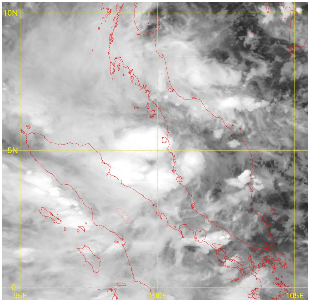
圖2.4 二零二五年十一月二十五日晚上8時左右熱帶氣旋森亞爾的紅外線衛星圖片，當時森亞爾在馬六甲海峽增強至熱帶風暴強度。
