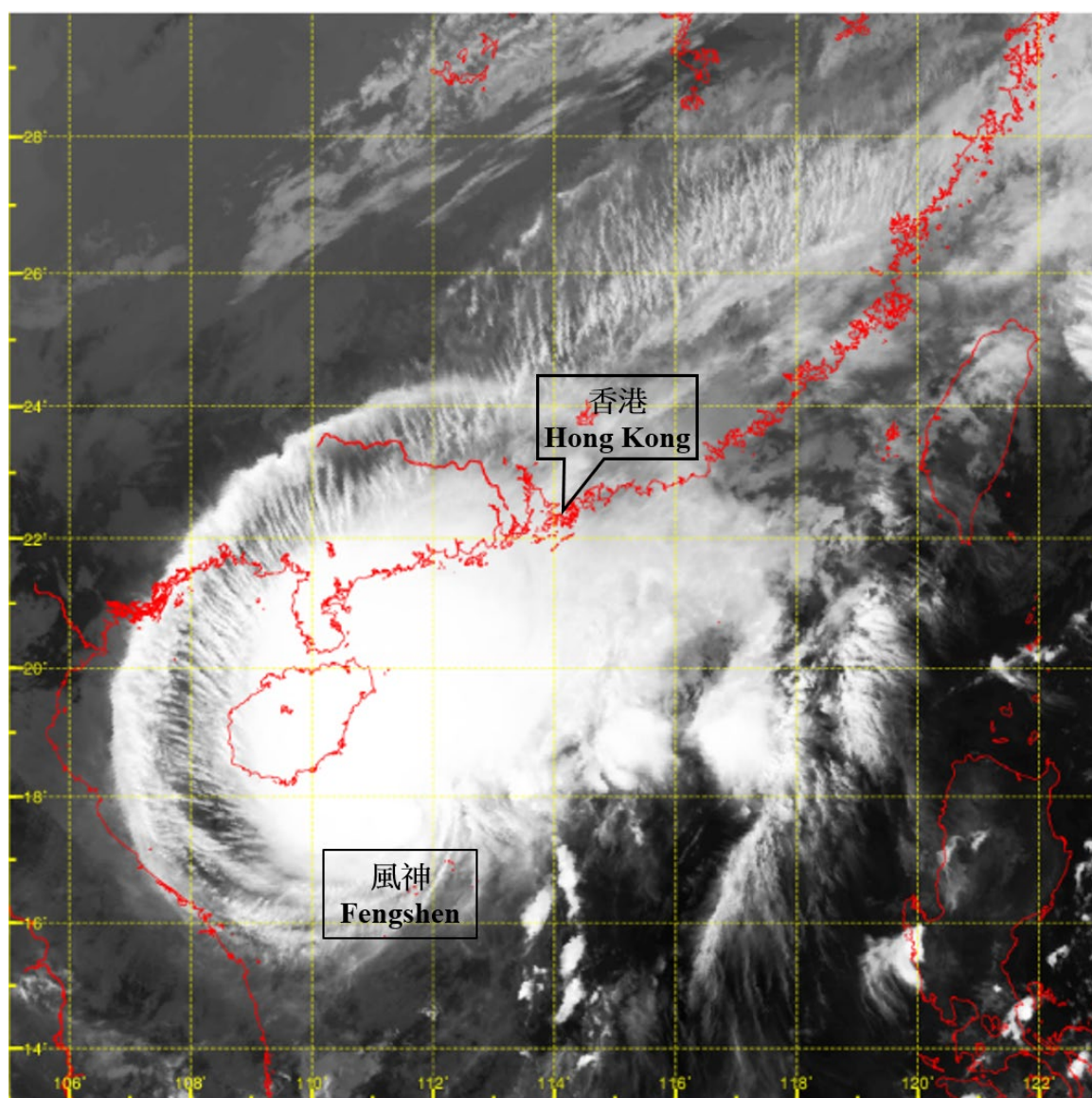
圖 3.13.3 二零二五年十月二十一日晚上 11 時左右的紅外線衛星圖片，當時風神達到其最高強度，中心附近最高持續風速估計為每小時 110 公里。
