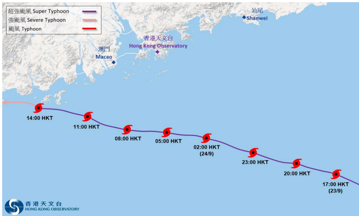
圖 3.11.1b 樺加沙(2518)接近香港時的路徑圖。
