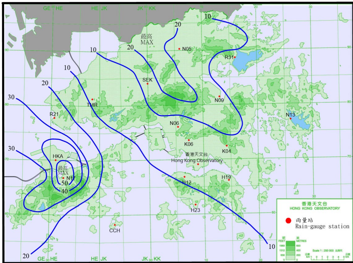
圖 3.12.2 二零二五年十月三日至五日的雨量分佈(等雨量線單位為毫米)。
