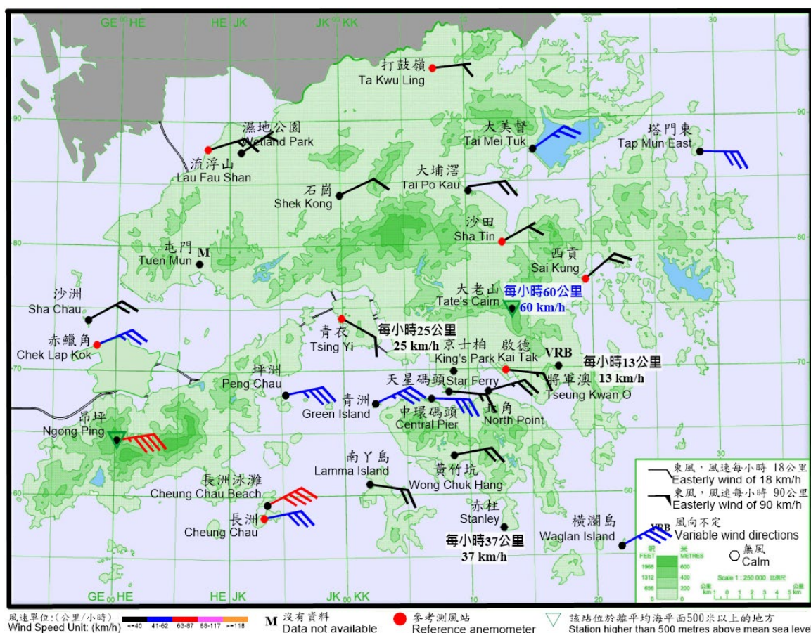
圖 3.12.3a 二零二五年十月四日下午8時05分香港各站錄得的十分鐘平均風向和風速。當時本港普遍吹強風程度的偏東風，包括香港國際機場、長洲、中環碼頭、橫瀾島及大老山。其中長洲泳灘及昂坪的風力更達烈風程度。
