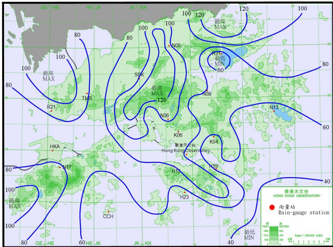
圖 3.1.2 二零二五年六月十一日至十五日的雨量分佈(等雨量線單位為毫米)。 Figure 3.1.2 Rainfall distribution on 11 – 15 June 2025 (isohyets are in millimetres).
