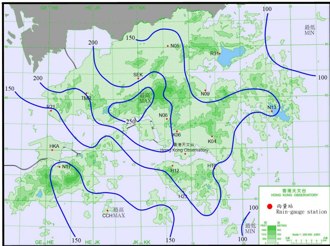
圖 3.3.4 二零二五年七月九日至十二日的雨量分佈(等雨量線單位為毫米)。 Figure 3.3.4 Rainfall distribution on 9 – 12 July 2025 (isohyets are in millimetres).
