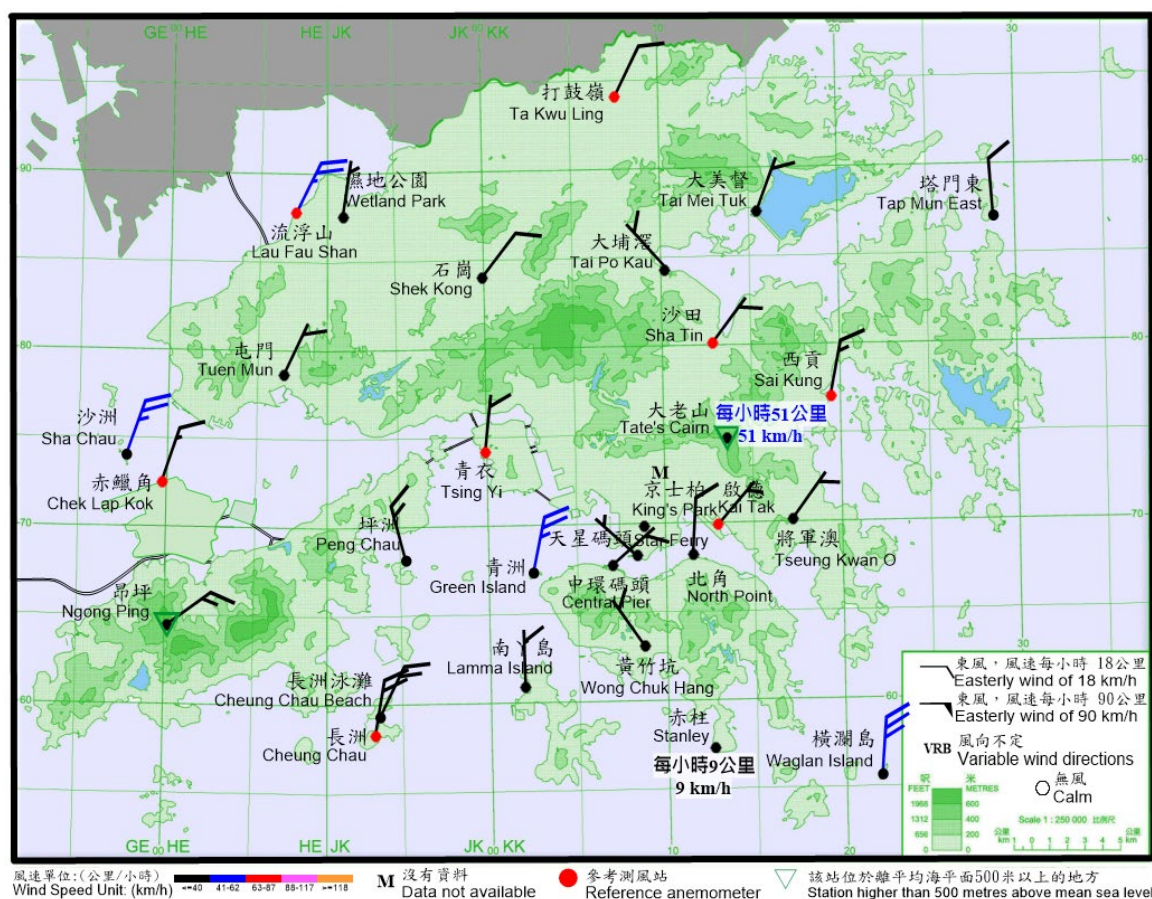
圖 3.13.2b 二零二五年十月二十一日下午12時40分香港各站錄得的十分鐘平均風向和風速。當時本港普遍吹北風，而流浮山、沙洲、青洲、橫瀾島及大老山的風力達到強風程度。
