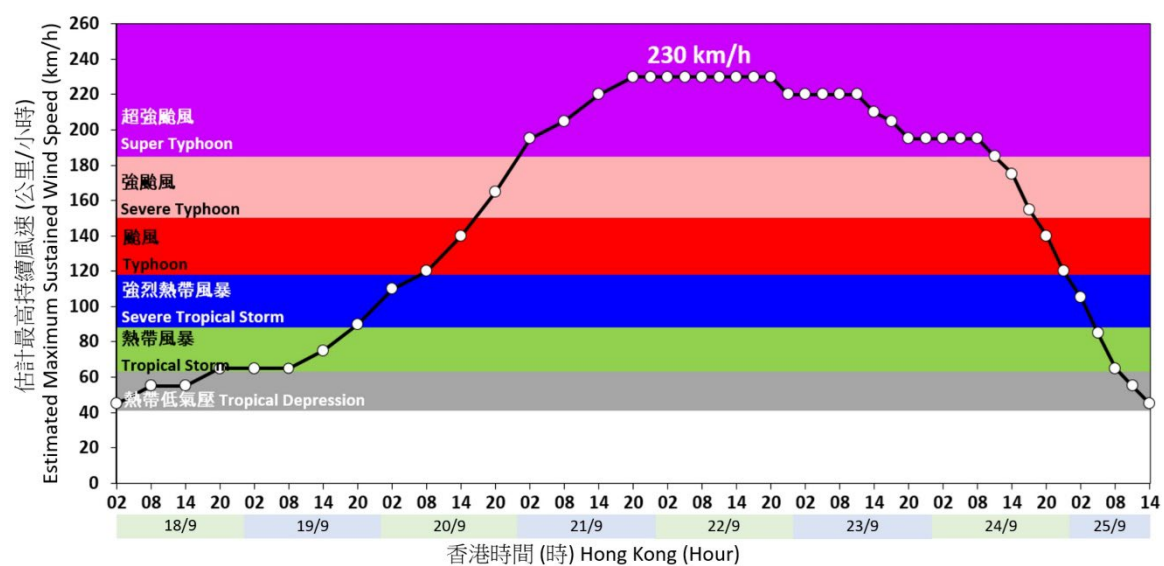
圖 3.11.2a 二零二五年九月十八日至二十五日樺加沙(2518)之估計最高持續風速的時間序列。
