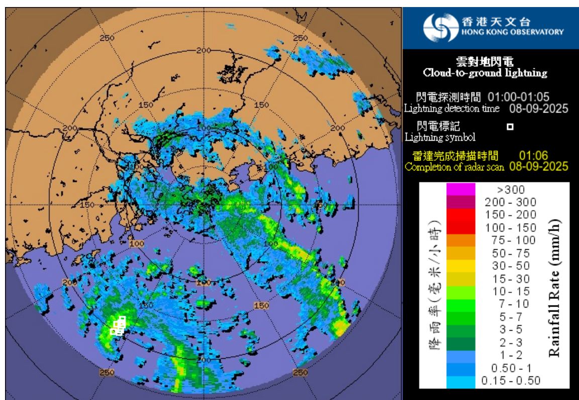
圖 3.9.7a 二零二五年九月八日上午1時06分的雷達回波與上午1時正至1時05分之間雲對地閃電位置的疊加圖像，顯示當時塔巴中心附近的對流強烈，並伴隨閃電。
