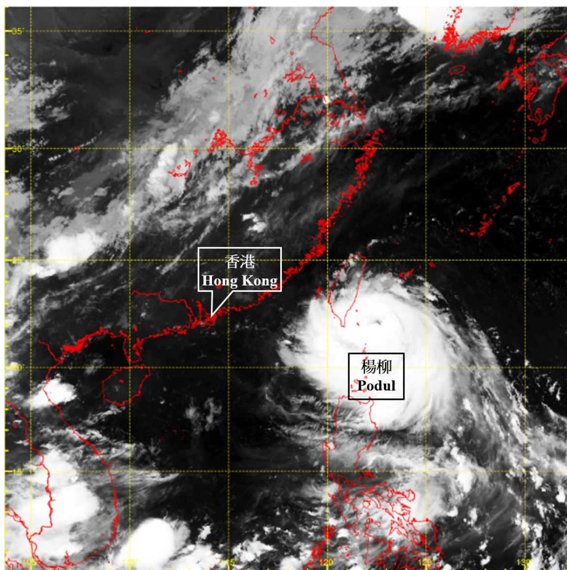
圖 3.5.3 二零二五年八月十三日早上 5 時左右的紅外線衛星圖片，當時楊柳迅速增強為強颱風，並達到其最高強度，中心附近最高持續風速估計為每小時 155 公里。
