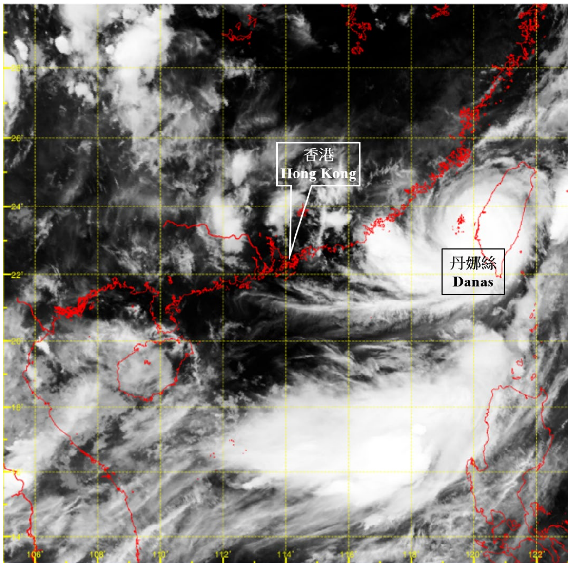
圖 3.3.2 二零二五年七月六日晚上 11 時左右的紅外線衛星圖片，當時丹娜絲在台灣西部沿岸迅速增強為強颱風，並達到其最高強度，中心附近最高持續風速估計為每小時 155 公里。
