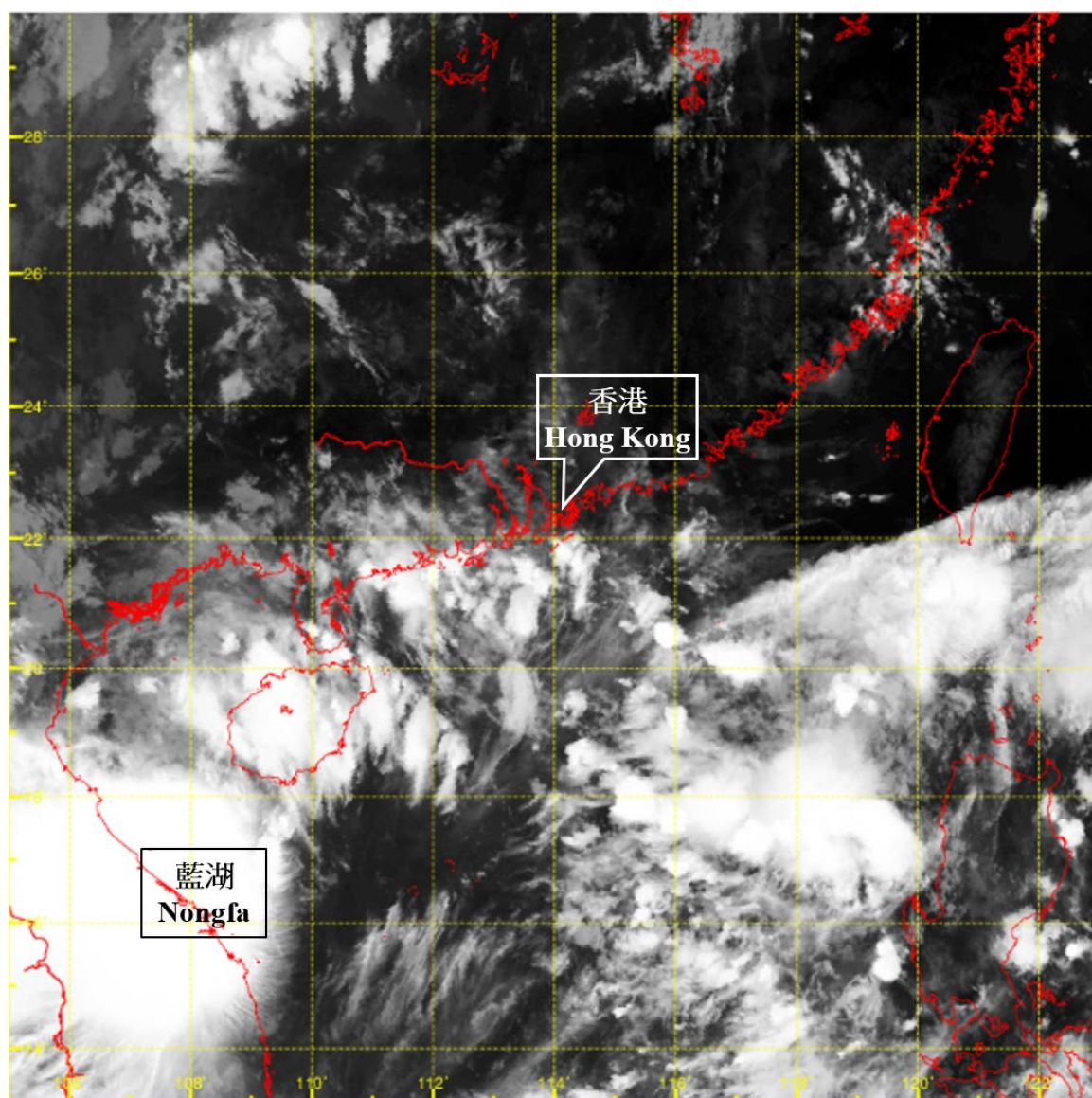
圖 3.8.2 二零二五年八月三十日早上 8 時左右的紅外線衛星圖片。當時藍湖在海南島西南海域增強為熱帶風暴，並達到其最高強度，中心附近最高持續風速估計為每小時 65 公里。
