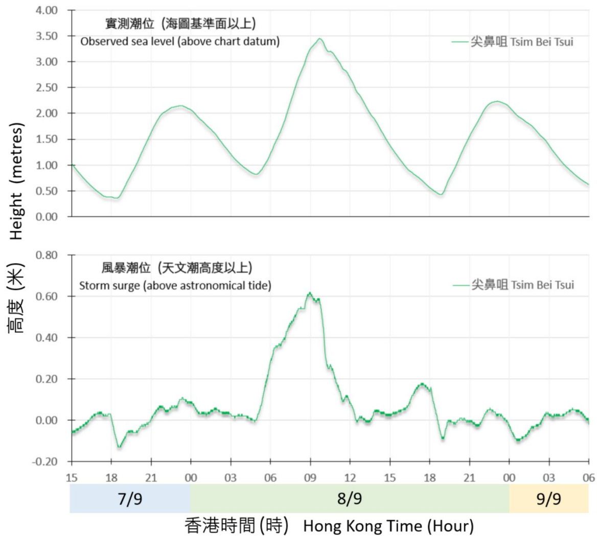
圖 3.9.5 二零二五年九月七日至九日尖鼻咀錄得的潮位(海圖基準面以上)及風暴潮(天文潮高度以上)。
