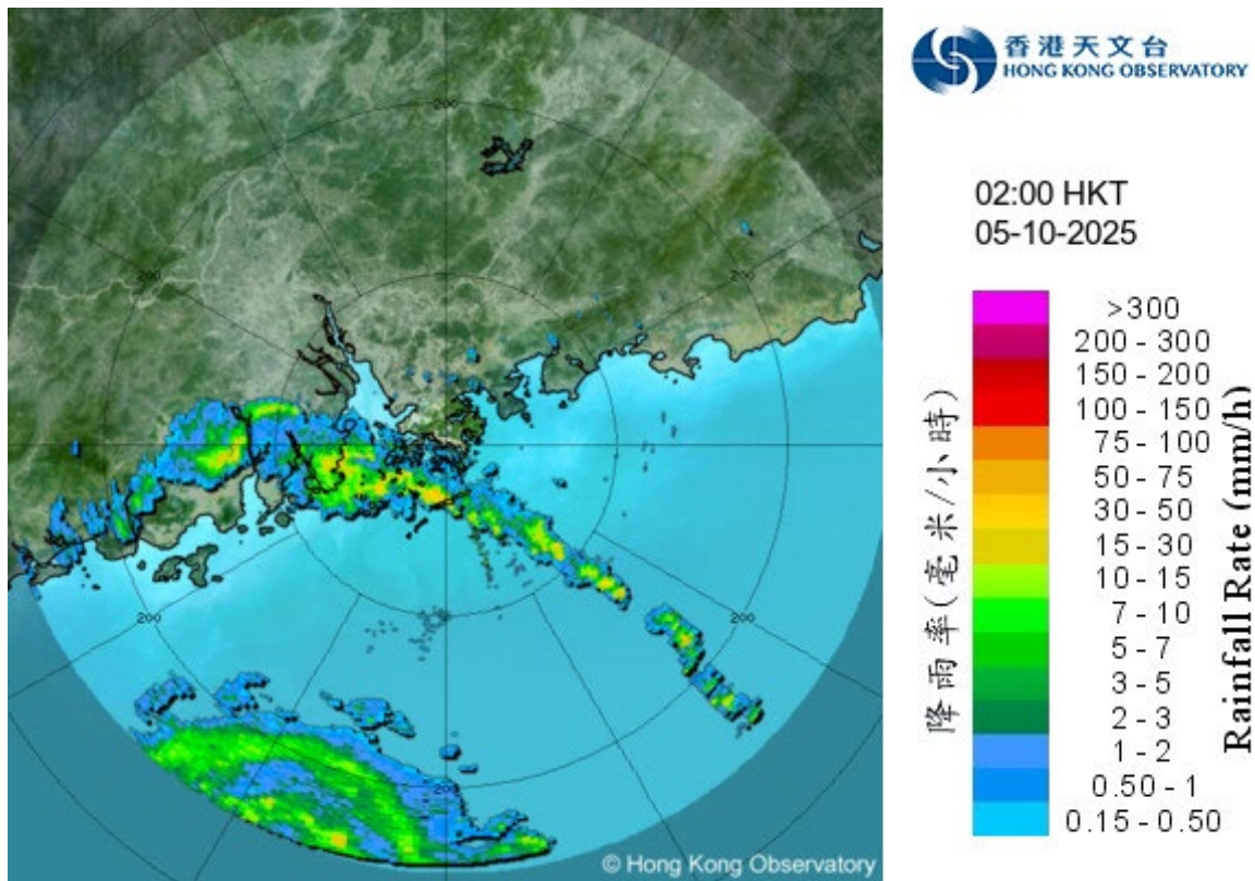
圖 3.12.5 二零二五年十月五日上午2時正的雷達回波圖像。當時麥德姆的中心位於香港之西南偏南約340公里。與其相關的外圍雨帶正影響珠江口一帶。
