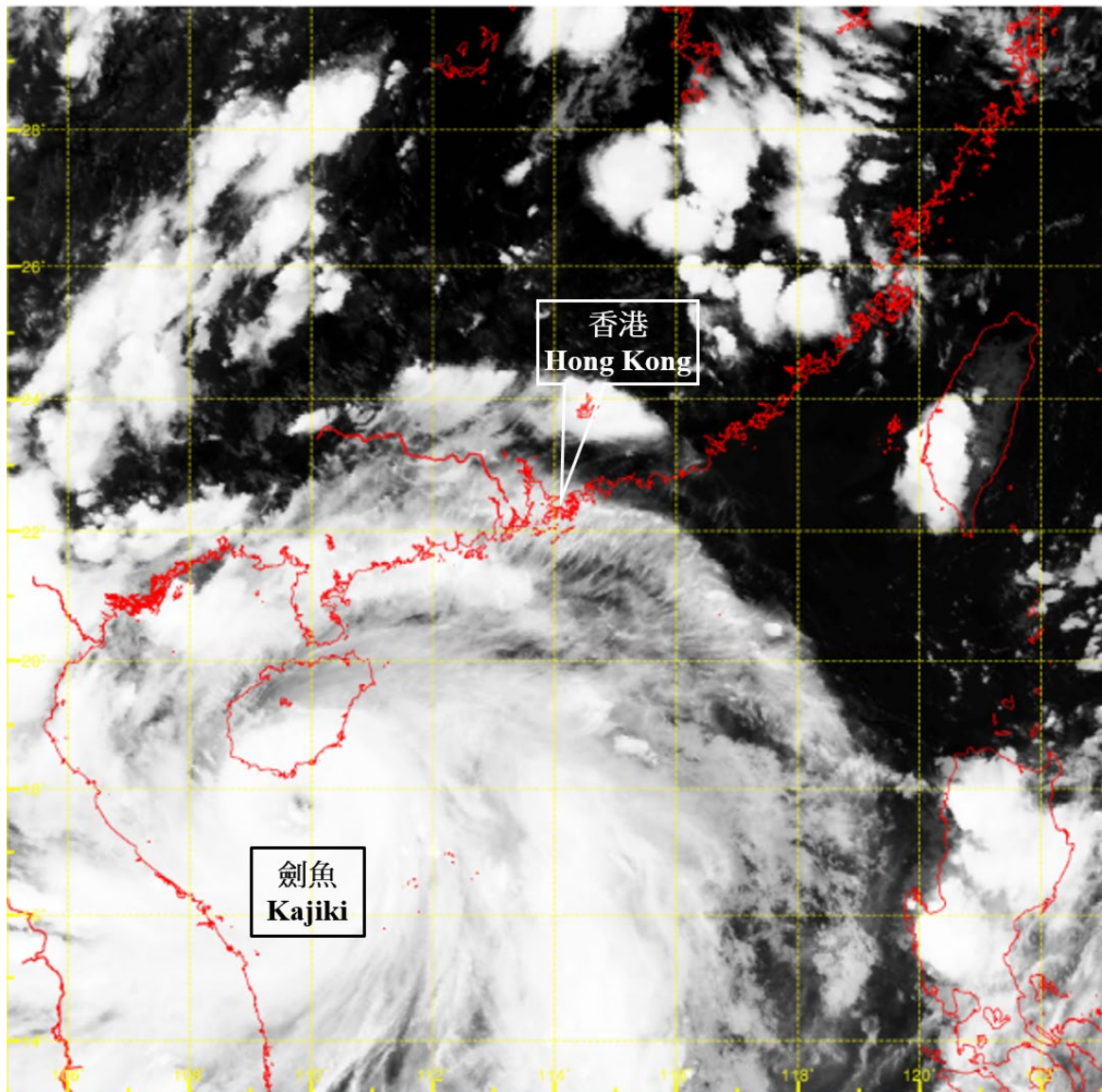
圖 3.7.2 二零二五年八月二十四日下午 5 時左右的紅外線衛星圖片，當時劍魚在海南島以南海域達到其最高強度，中心附近最高持續風速估計為每小時 175 公里。
