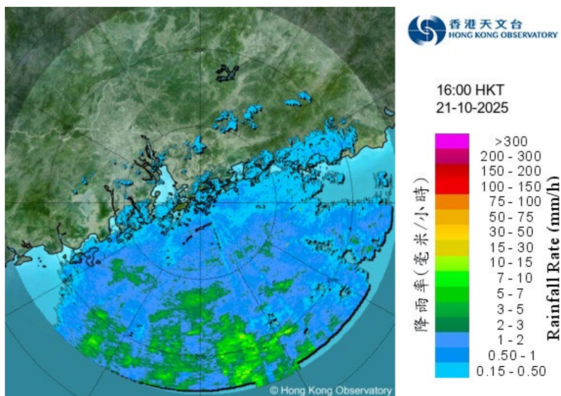
圖 3.13.4 二零二五年十月二十一日下午4時正的雷達回波圖像。與風神相關的雨區持續影響南海北部，但受較乾燥的東北季候風影響，雨區靠近廣東沿岸時有所減弱。
