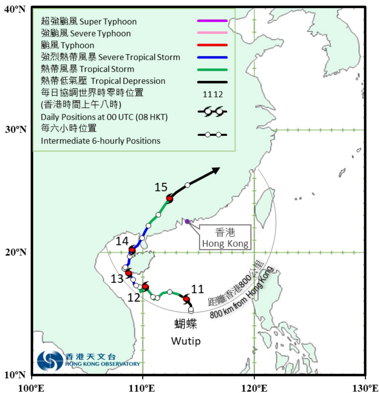
圖 3.1.1 二零二五年六月十日至十五日蝴蝶(2501)的路徑圖。
