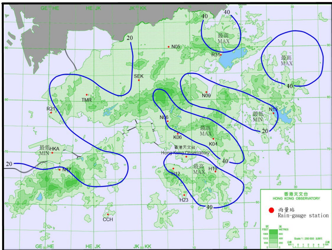
圖 3.6.2 二零二五年八月十六日至十七日的雨量分佈(等雨量線單位為毫米)。 Figure 3.6.2 Rainfall distribution on 16 – 17 August 2025 (isohyets are in millimetres).
