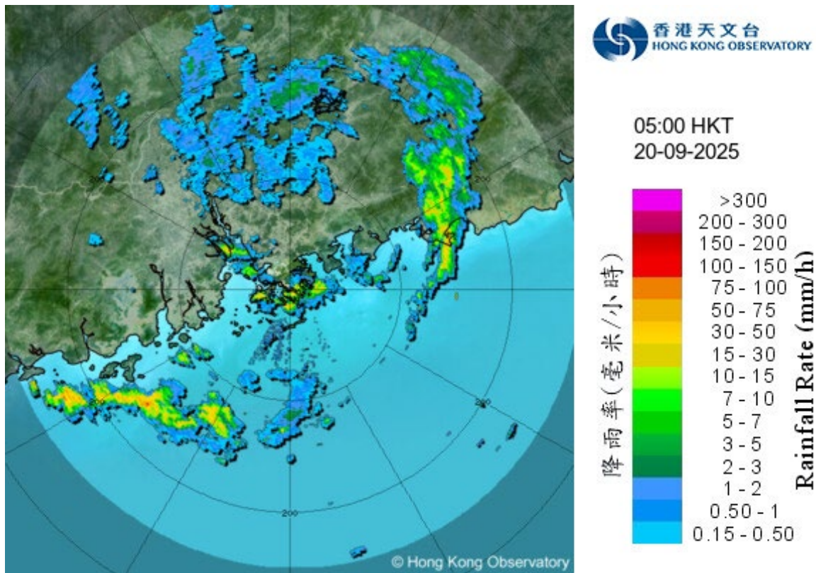
圖 3.10.5 二零二五年九月二十日上午5時正的雷達回波圖像。當時米娜的中心位於廣東惠州，與其相關的強雨帶正影響本港，黃色暴雨警告正在生效。
