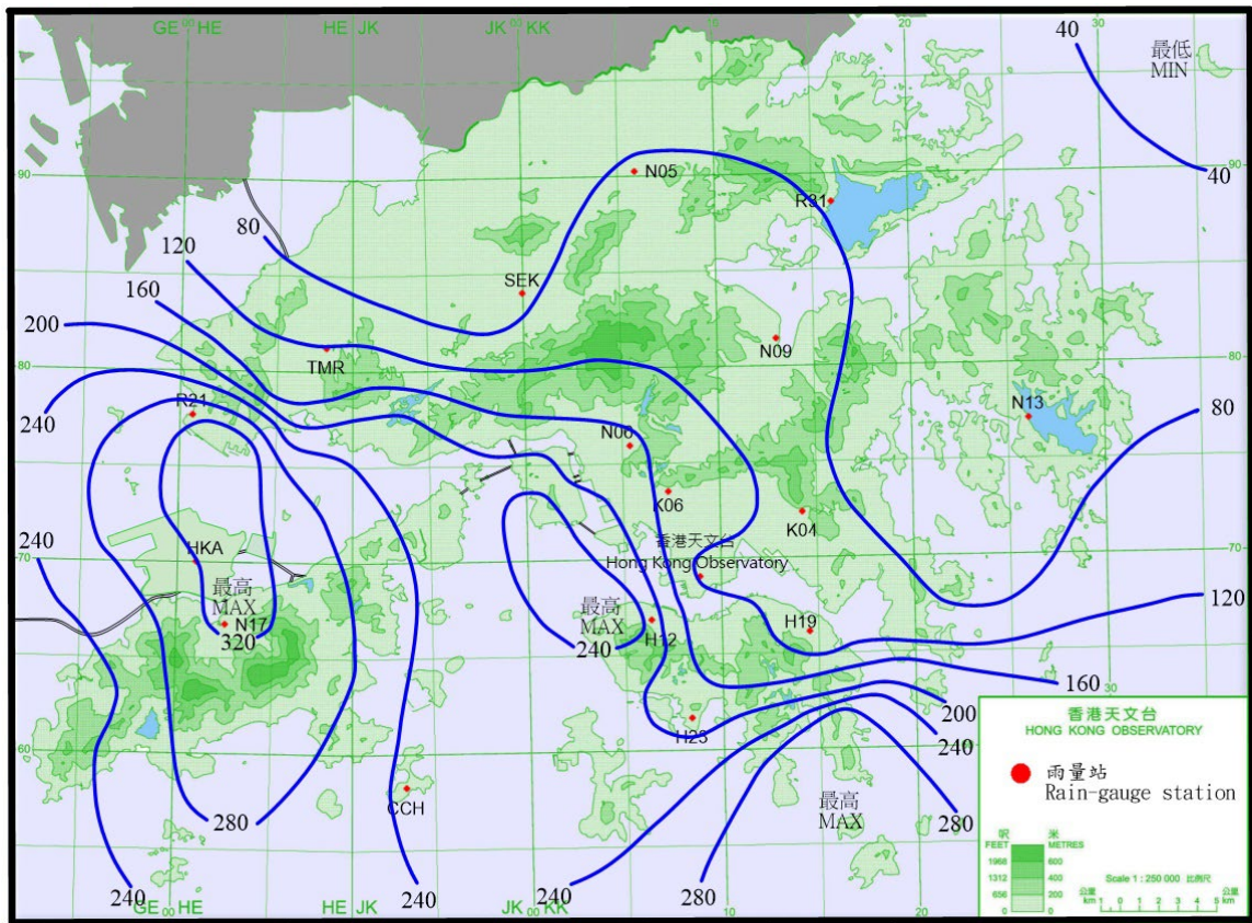
圖 3.5.2 二零二五年八月十三日至十四日的雨量分佈(等雨量線單位為毫米)。
