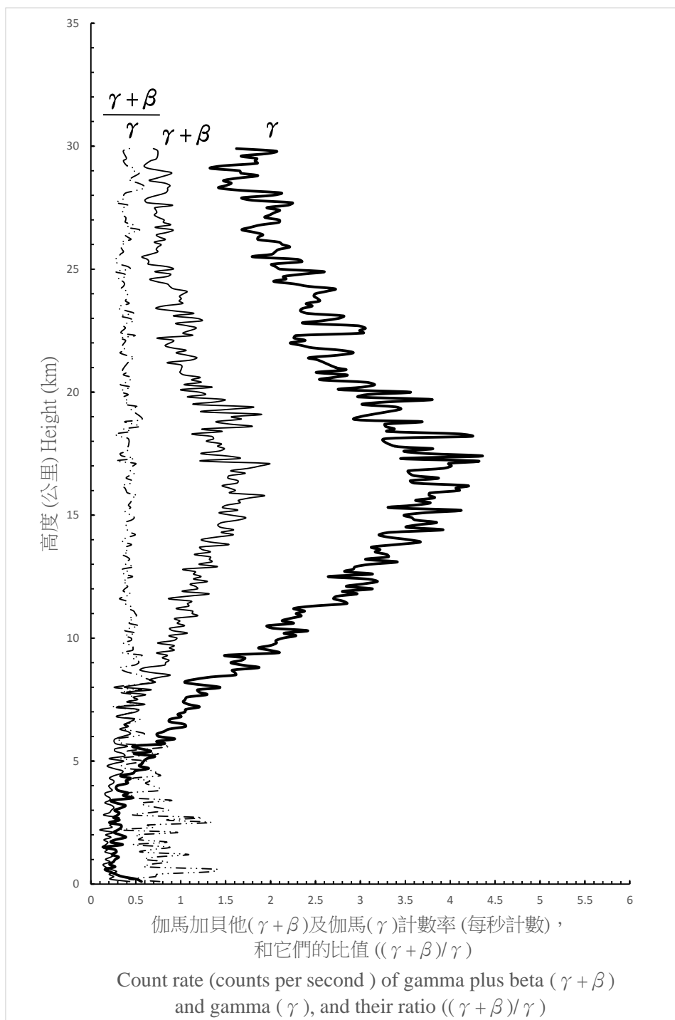
圖 6. 二零一五年內在京士柏進行的高空輻射探測之平均大氣放射性垂直廓線(探測日期為：四月二十日、六月四日、十二月三日、十二月十五日)。
