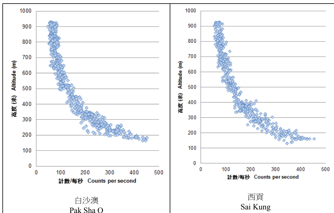
圖 5. 空中輻射監測系統在白沙澳及西貢上空測量到的計數率隨高度的變化(二零一四年十月二十日)。
