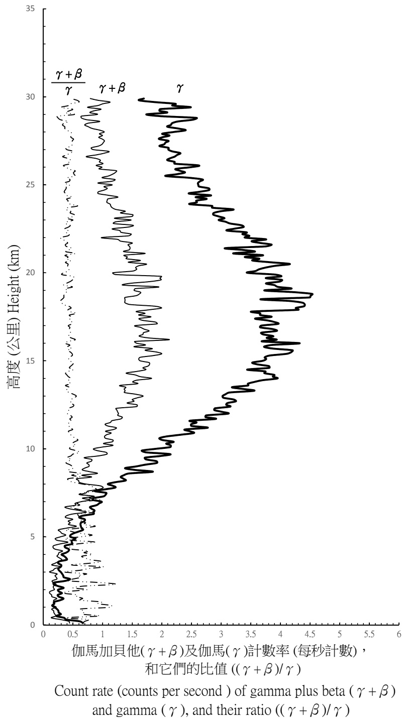
圖 7. 二零一四年內在京士柏進行的高空輻射探測之平均大氣放射性垂直廓線 (探測日期為: 三月二十七日、七月三十一日、九月四日、十二月二十二日)。
