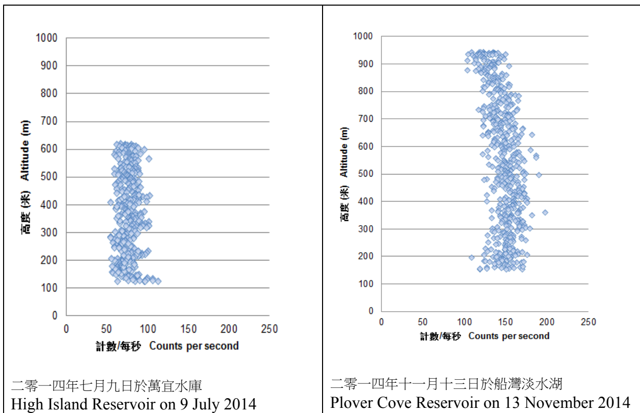
圖 6. 空中輻射監測系統在二零一四年於萬宜水庫和船灣淡水湖水面上空測量到的計數率隨高度的變化。
