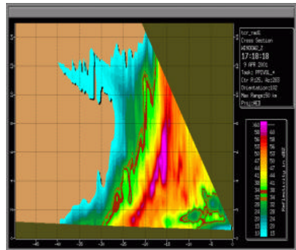
(d) Vertical section along X - Y for (c)
