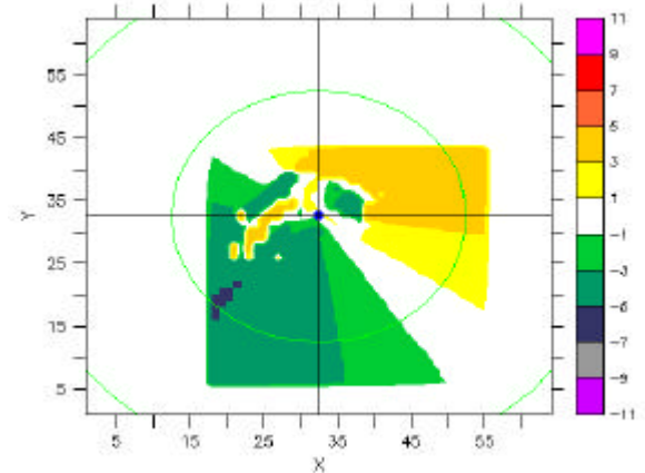
(d) 3-km level computed Doppler field
