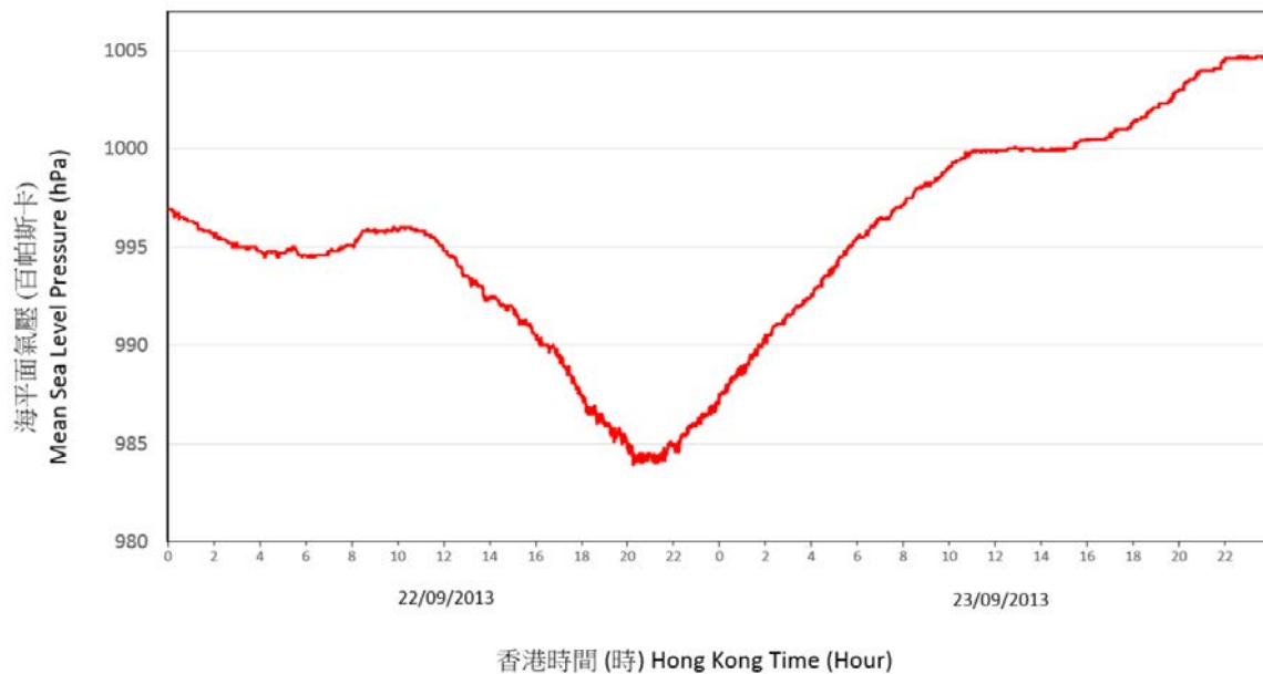
圖 3.6.4b 二零一三年九月二十二日至二十三日橫瀾島自動氣象站錄得的海平面氣壓。
