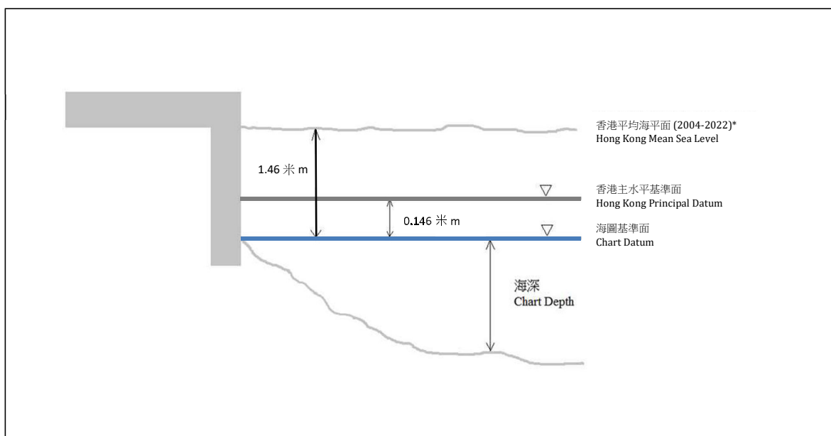
香港高程基準示意圖
