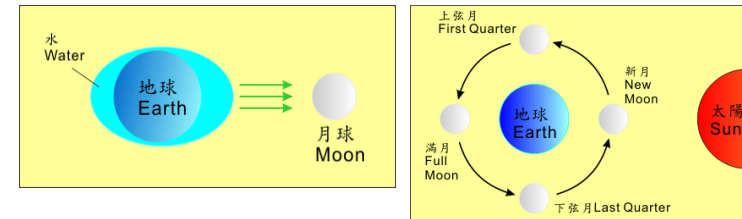
潮汐的示意圖 (不依比例)
